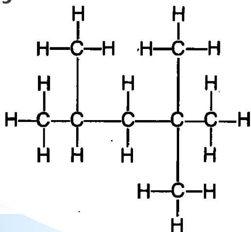
Iso-Octane
