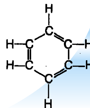
Benzene
